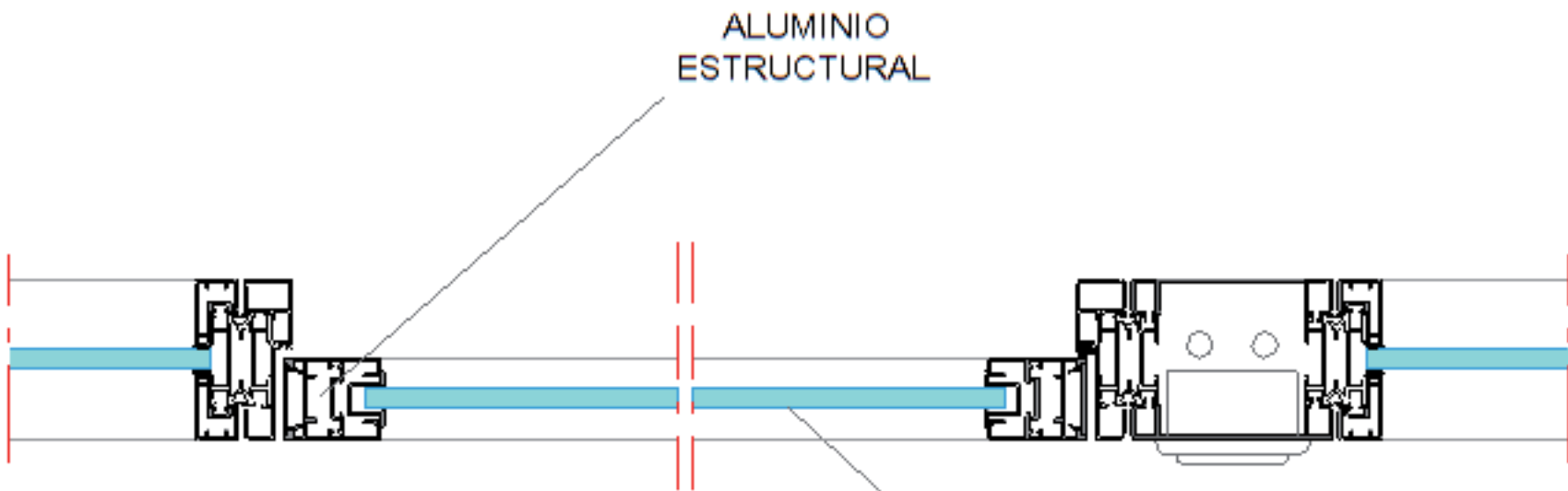
SECCION VERTICAL
