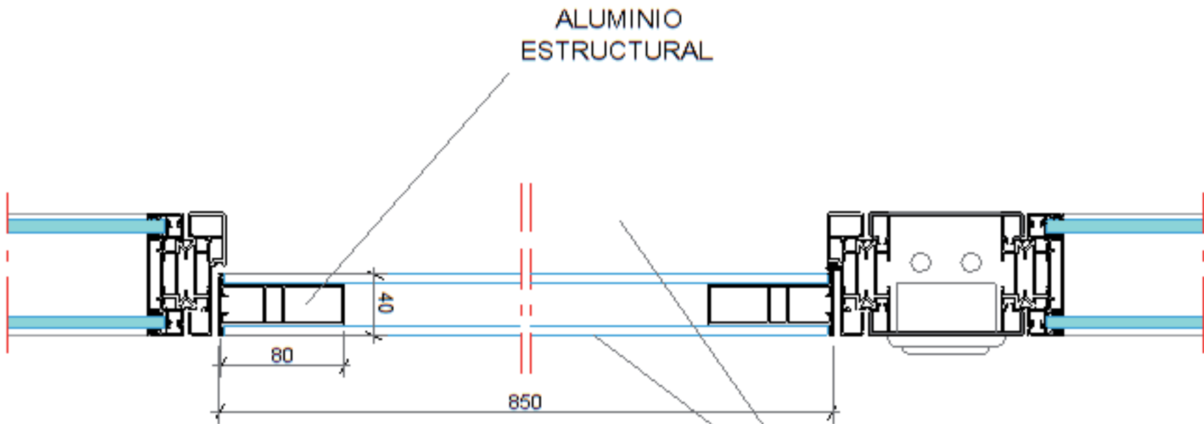
SECCION VERTICAL
