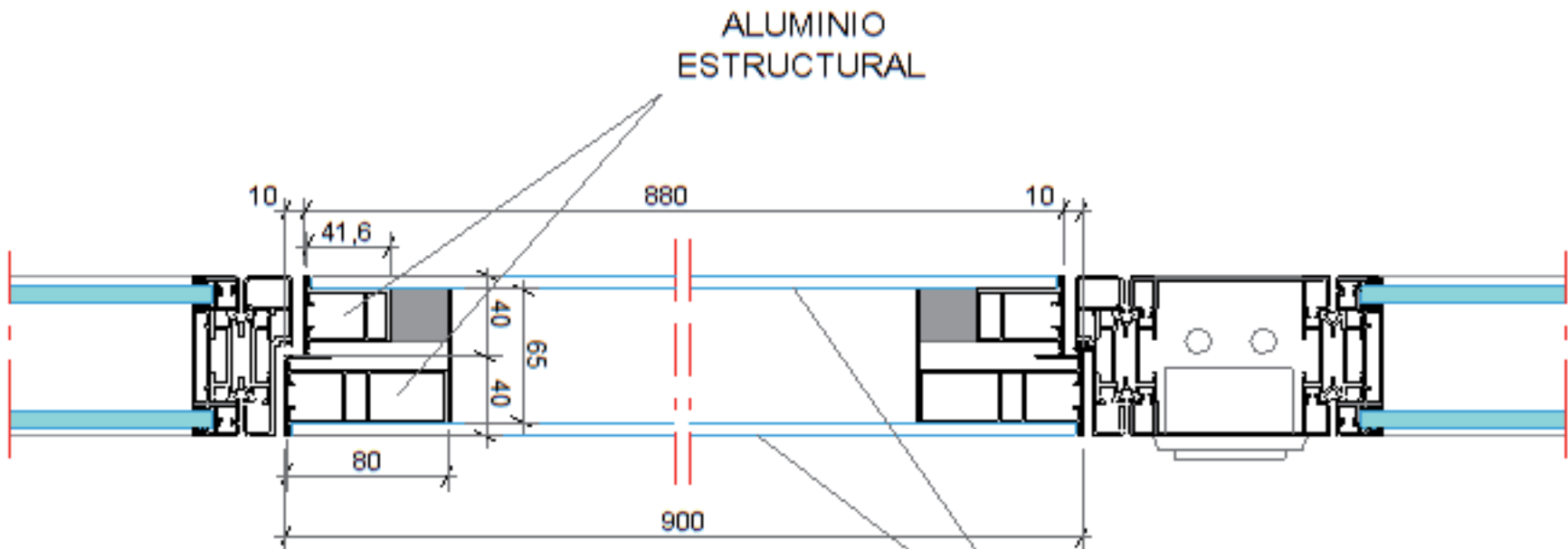
SECCION VERTICAL
