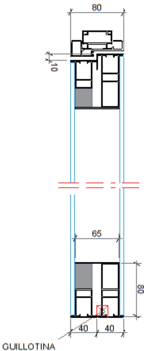
SECCION VERTICAL
