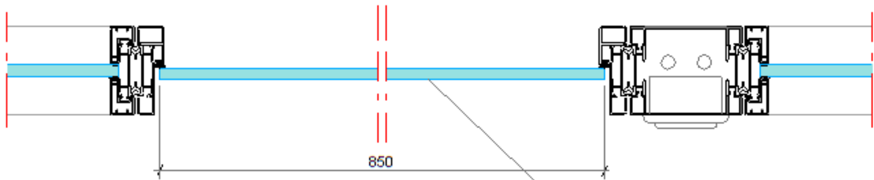
SECCION HORIZONTAL
