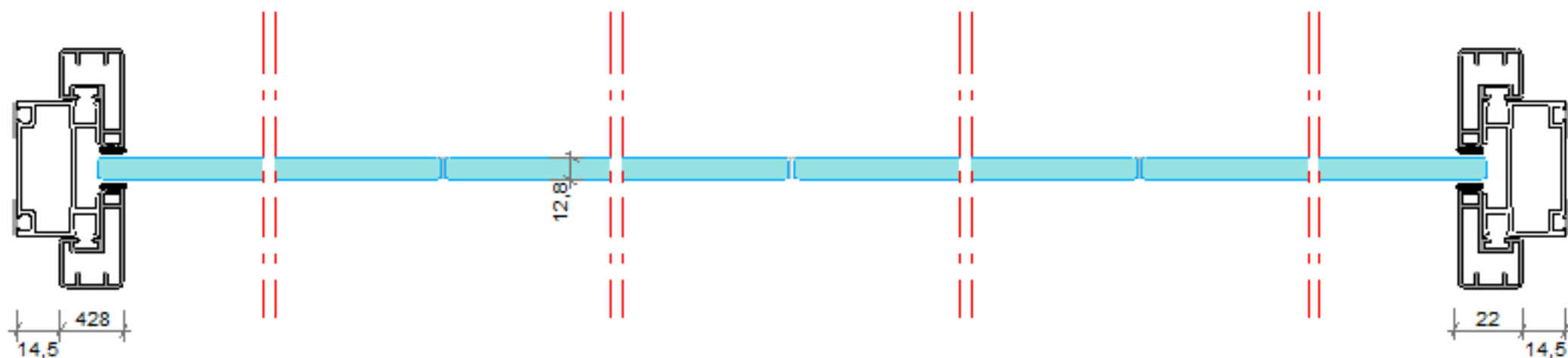
SECCION HORIZONTAL
