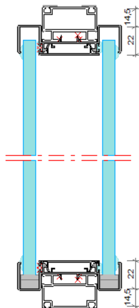
SECCION VERTICAL
